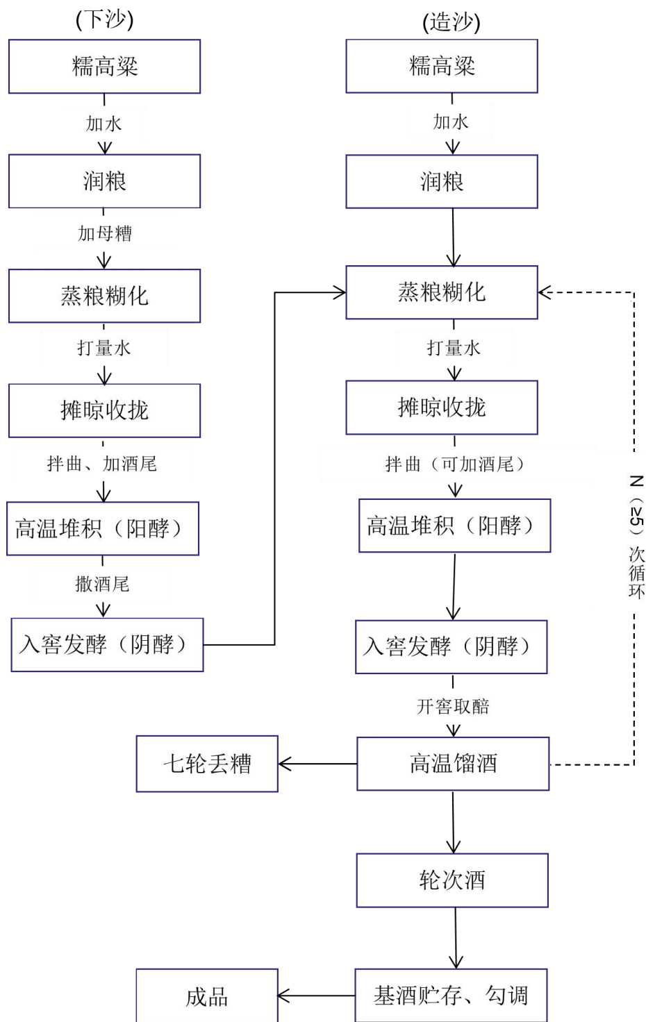
图A.1 咖啡风味酱香型白酒（高温大曲）主要生产流程示例图
